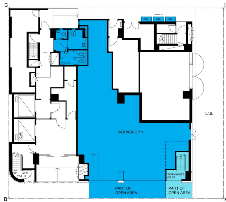
G/F PLAN
