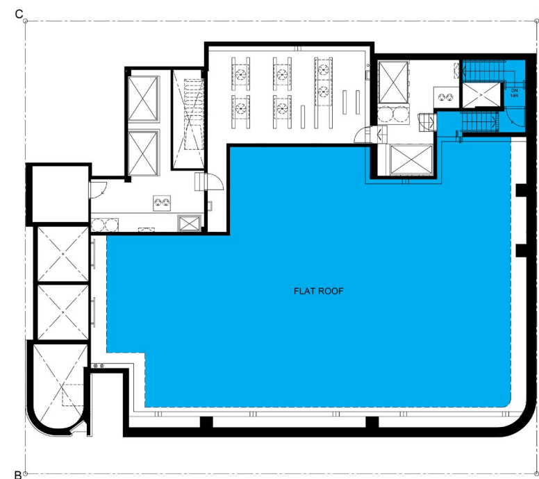
R/F PLAN
