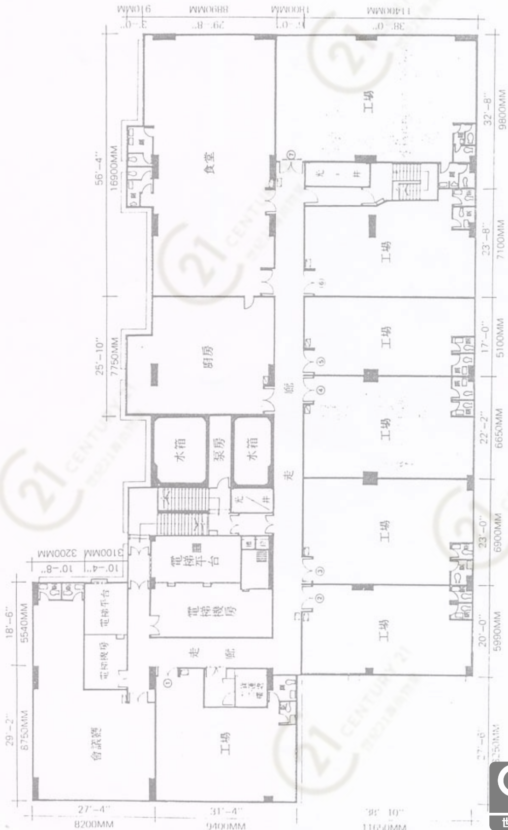
十二樓平面圖 12th Floor Plan
