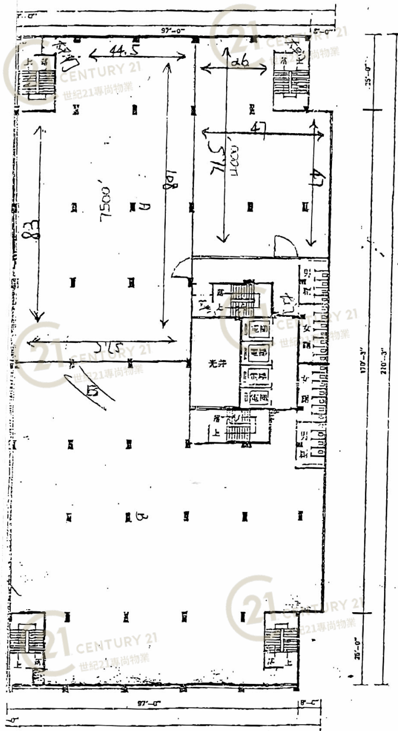
三樓至十二樓平面圖
