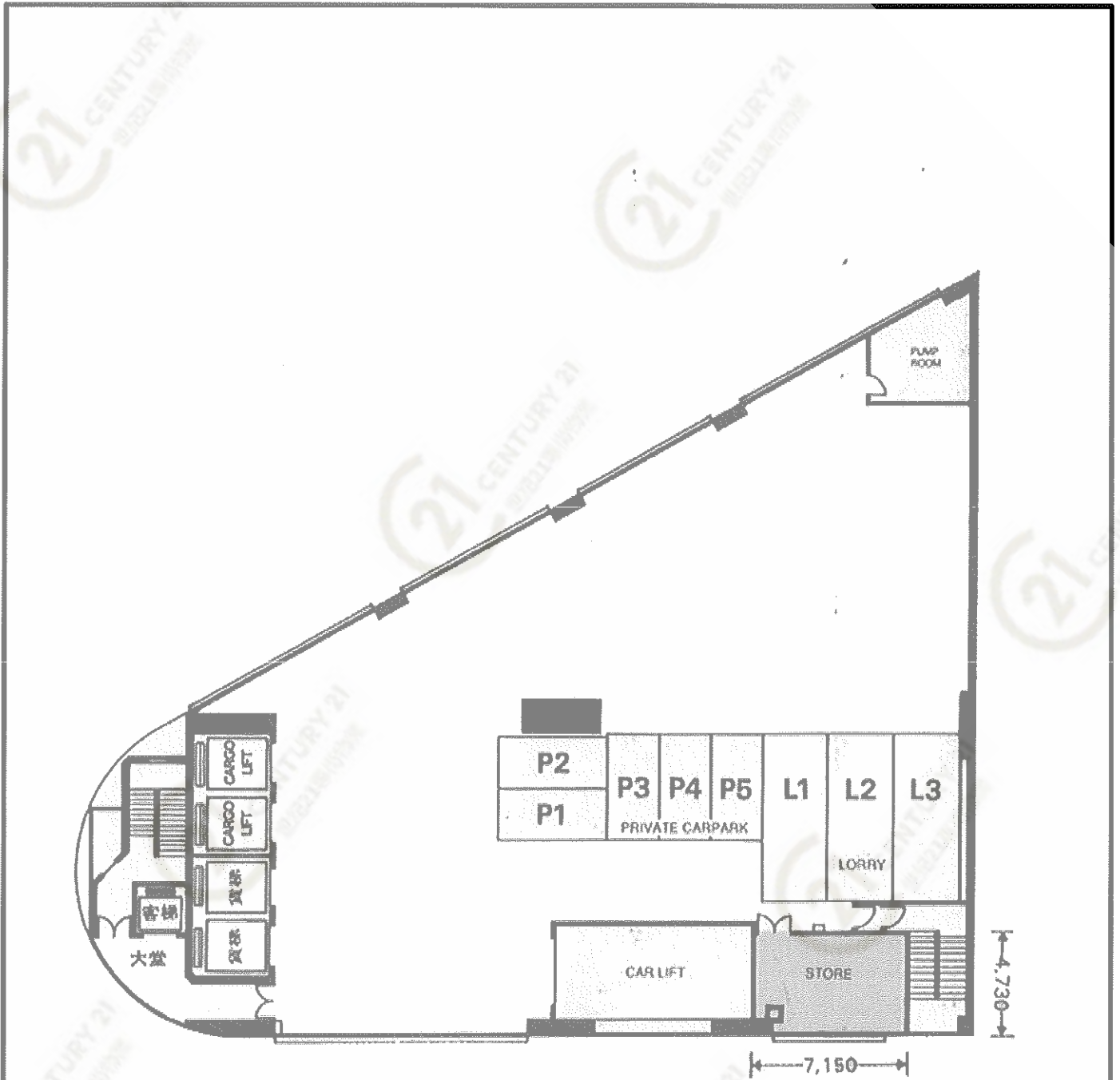
2ND FLOOR PLAN 二樓
