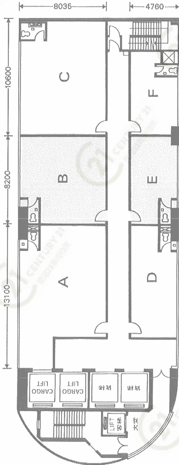
TYPICAL FLOOR PLAN (20TH - 25 TH FLOOR) 大廈平面圖(二十至二十五樓)
